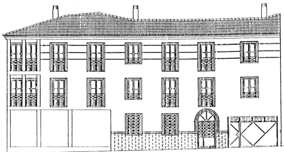
ALZADO CALLE CACHORRO
