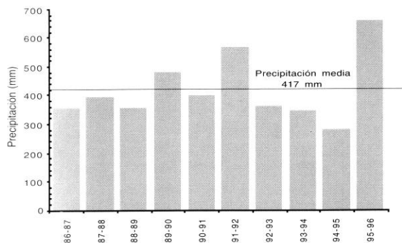
Fig. 1. Precipitaciones durante 1986-1996.
