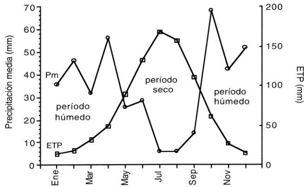
Fig. 3. Distribución de los periodos secos y húmedos
