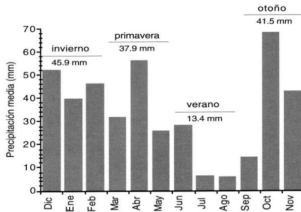
Fig. 2. Precipitación media en los diferentes meses del año.
